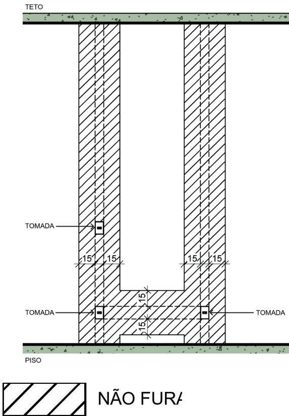
Figura 74 Desenho esquemático indicando faixa de parede que NÃO pode ser perfurada
