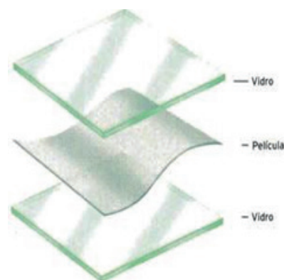
Figura 39 Camadas do vidro laminado
