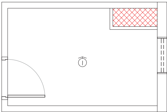
PLANTA BAIXA - BANH SOCIAL ESC.: 1/25
