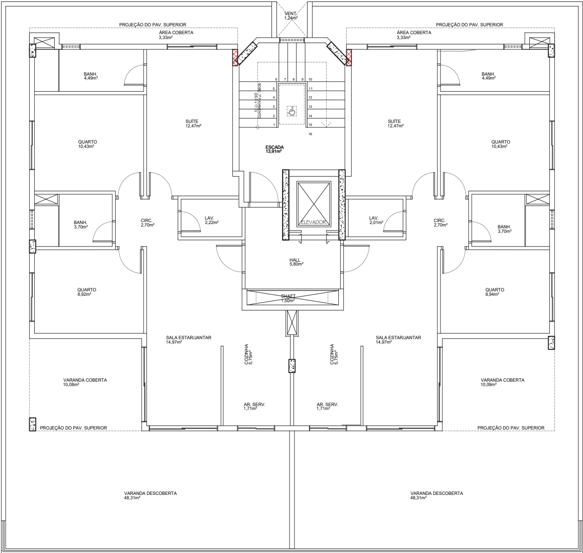
PLANTA BAIXA - PRUMADA DRENO AR COND - 6º PAVIMENTO ESC.: 1/50
