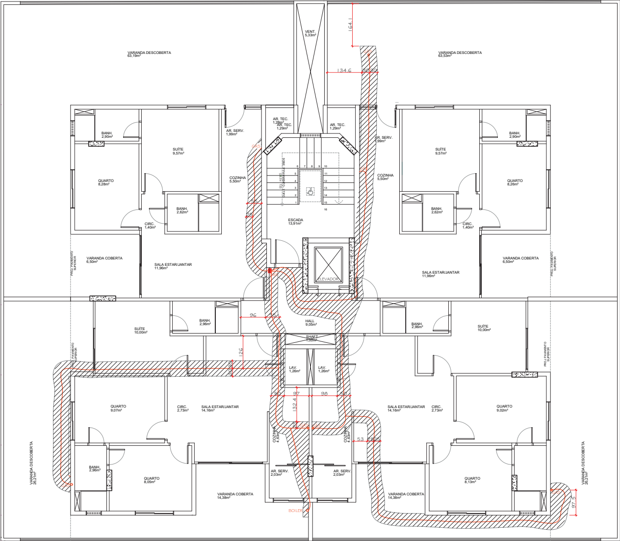
PLANTA BAIXA - TUBULAÇÃO DE GÁS - 2º PAVIMENTO ESC.: 1/50
