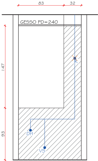
VISTA 01 - LAVABO ESC.: 1/25
