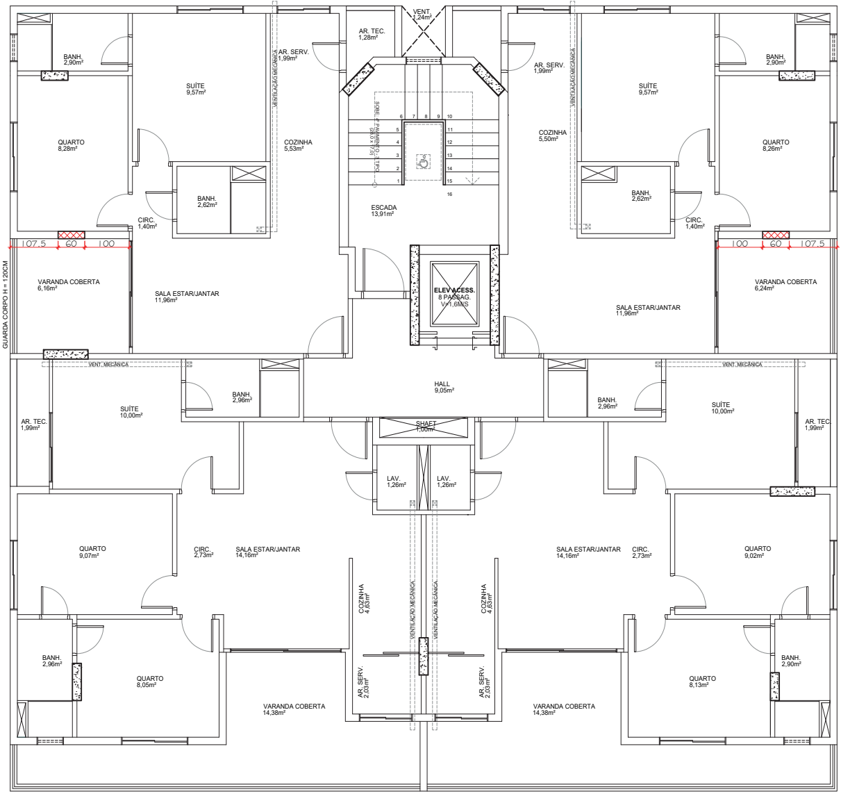
PLANTA BAIXA - PRUMADA DE AR COND. - 3º PAVIMENTO ESC.: 1/50
