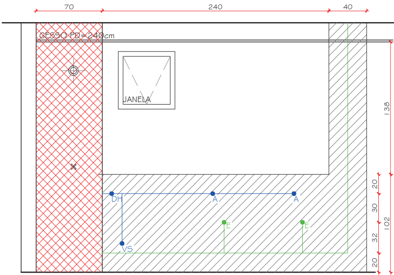
VISTA 01 - BANH. SUÍTE ESC.: 1/25
