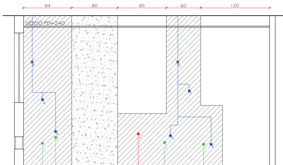
VISTA O1 - COZINHA ESC.: 1/25
