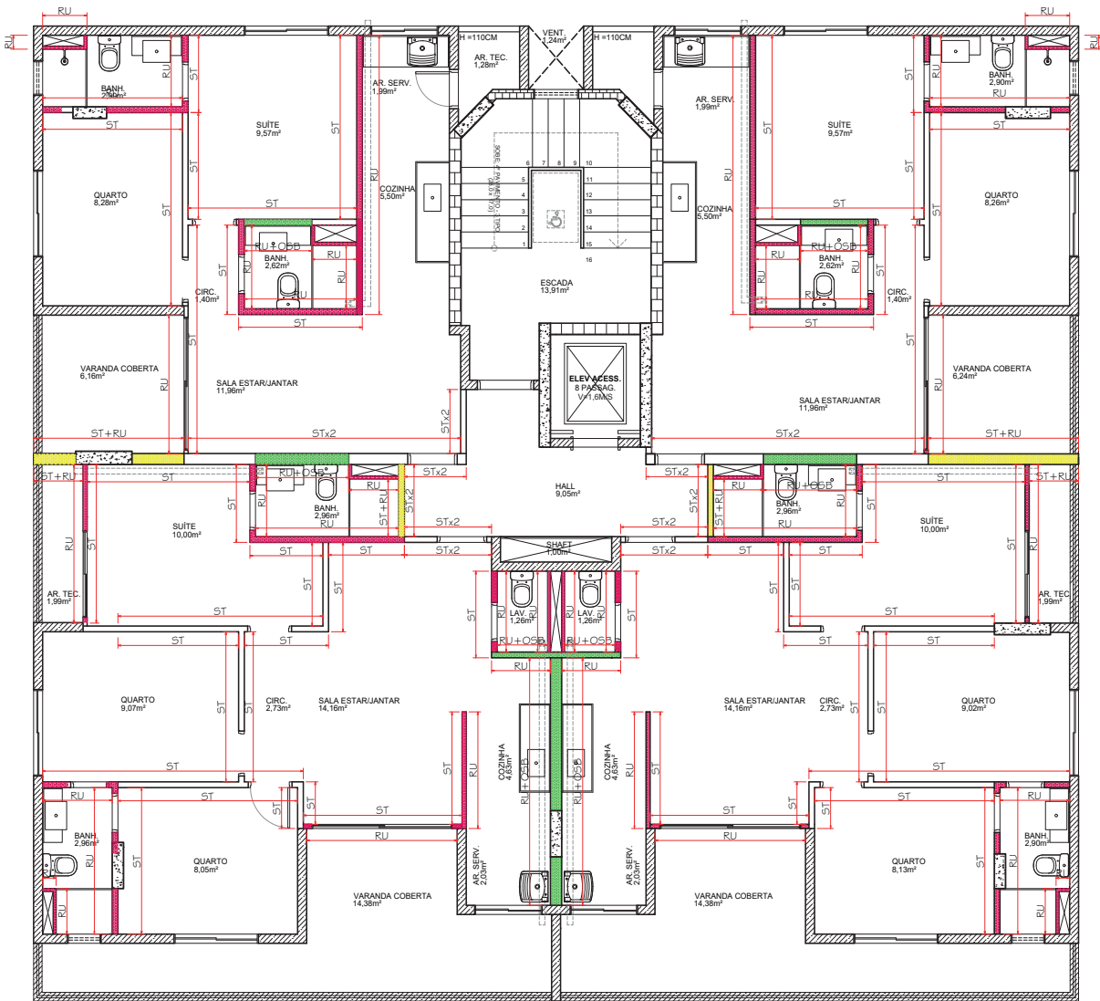
PLANTA BAIXA - DRYWALL - PAVIMENTO TIPO (2º AO 5º PAV.) E.C.: 1/50
