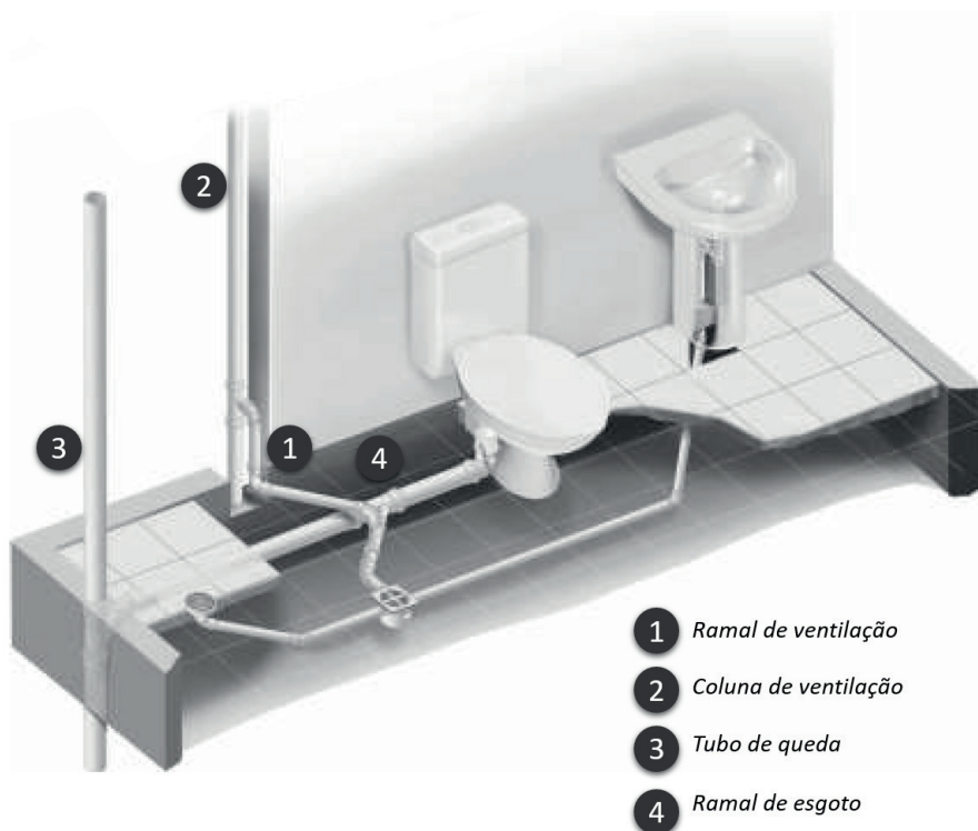
Figura 55 Representação da tubulação de esgoto de um banheiro
