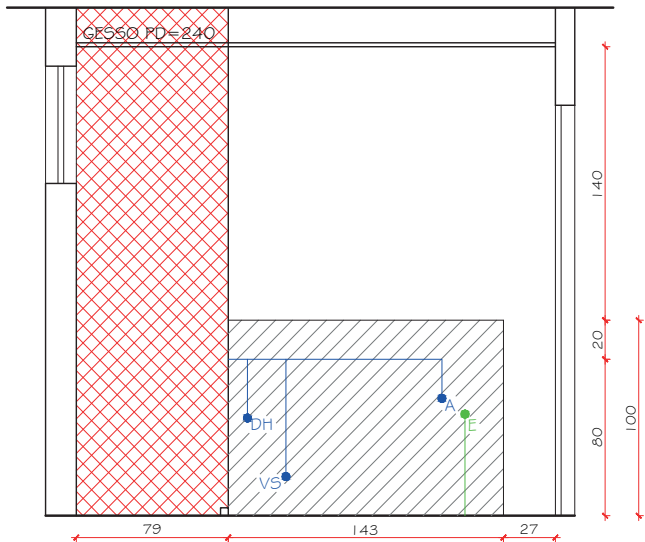
VISTA O1 - BANH SUITE ESC.: 1/25
