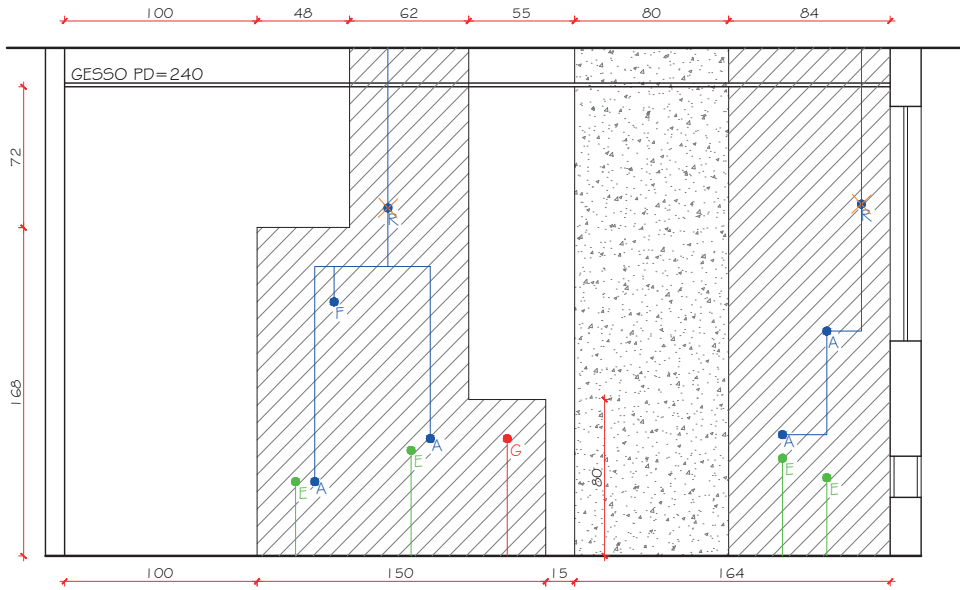
VISTA O.I - COZINHA ESC.: 1/25
