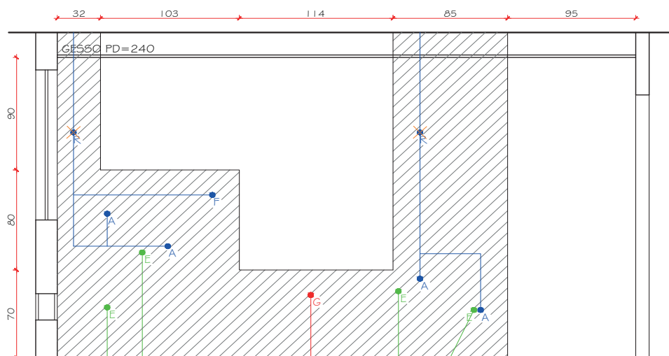
VISTA 01 - COZINHA ESC.: 1/25
