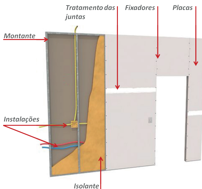
Figura 7 Componentes da parede de Drywall
