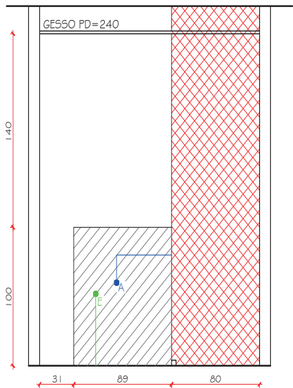
VISTA 01 - BANH SOCIAL ESC.: 1/25
