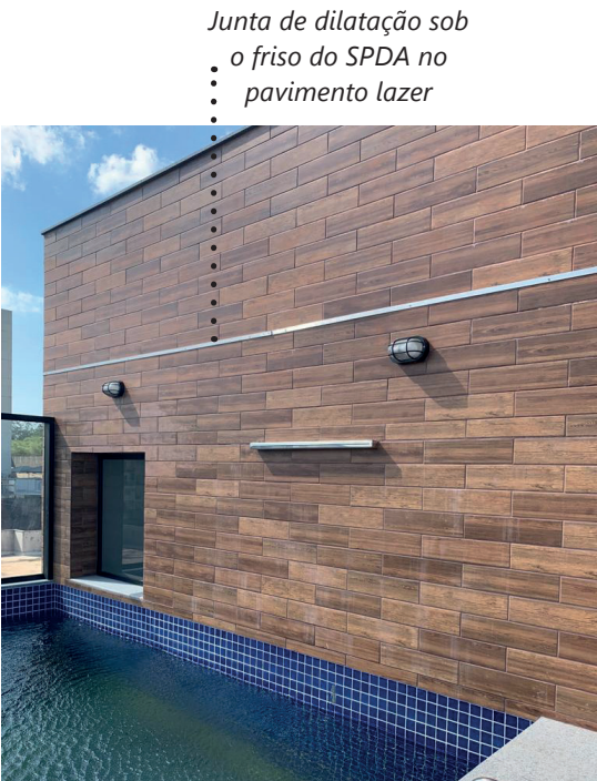
Figura 25 Junta de dilatação na fachada
