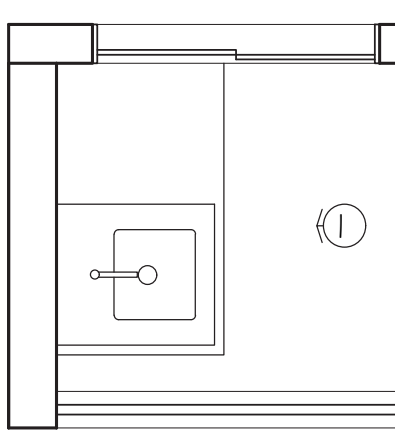
PLANTA BAIXA - VARANDA ESC.: 1/25
