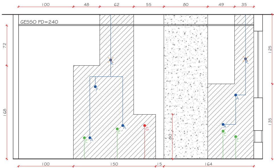
VISTA 01 - COZINHA ESC.: 1/25
