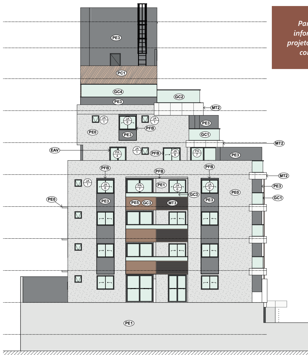
Figura 21 Fachada do Edifício Roof Top com aplicação de Textura e Revestimentos
