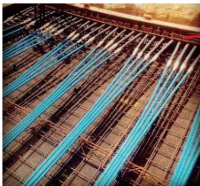
Figura 2 Exemplo de Cordoalhas
