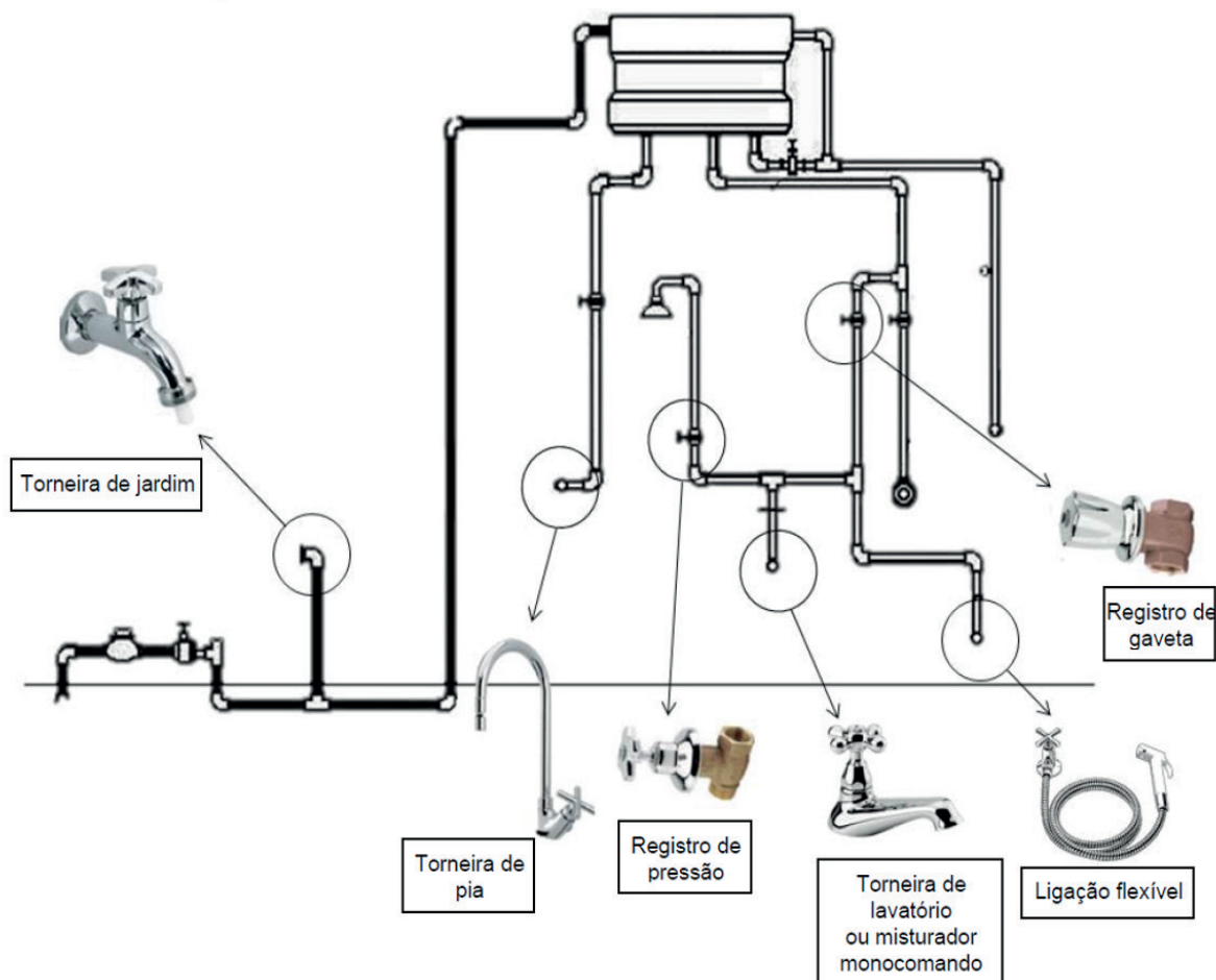
Figura 64 Identificação e posicionamento dos principais metais sanitários
