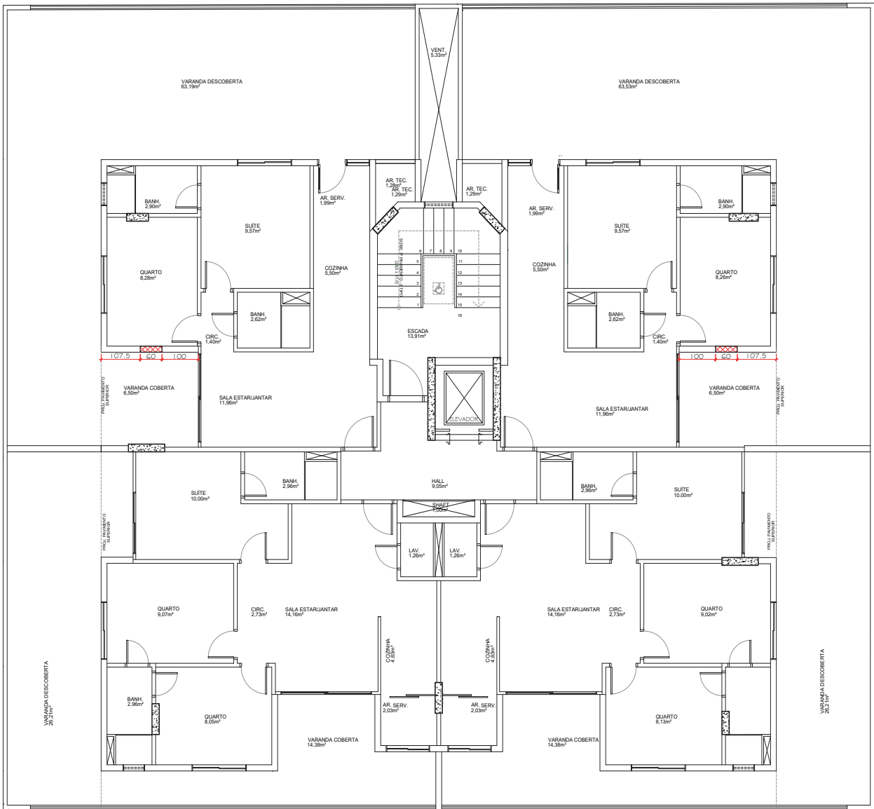
PLANTA BAIXA - PRUMADA DE AR COND. - 2º PAVIMENTO ESC.: 1/50
