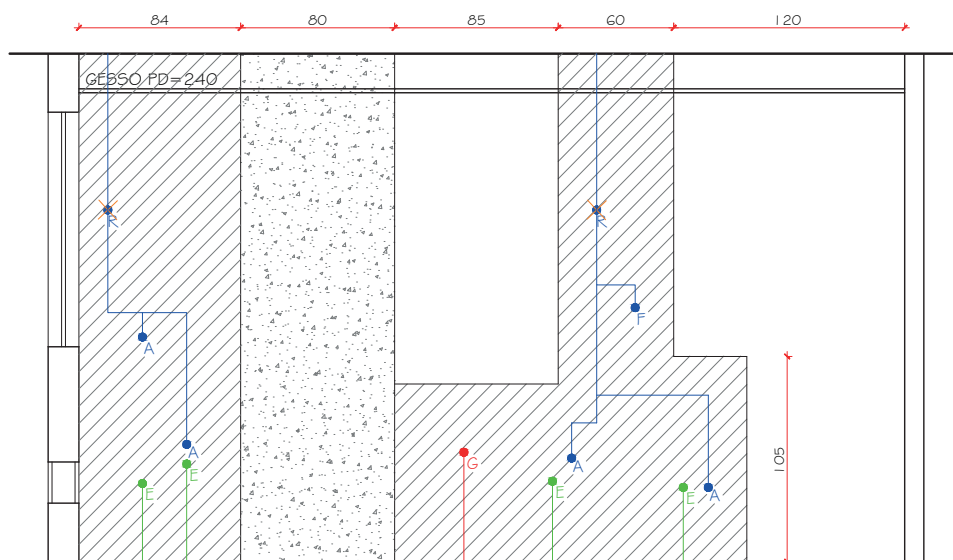
VISTA 01 - COZINHA ESC.: 1/25
