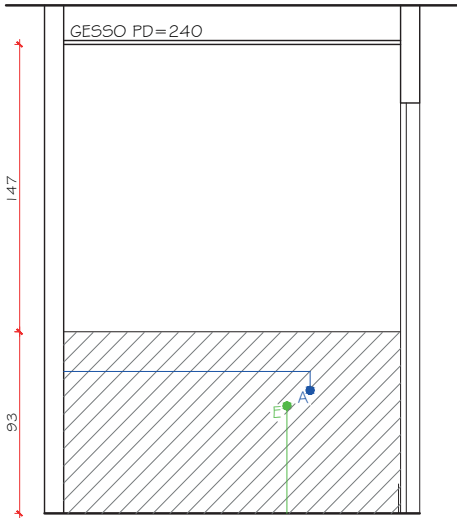
VISTA 02 - LAVABO ESC.: 1/25
