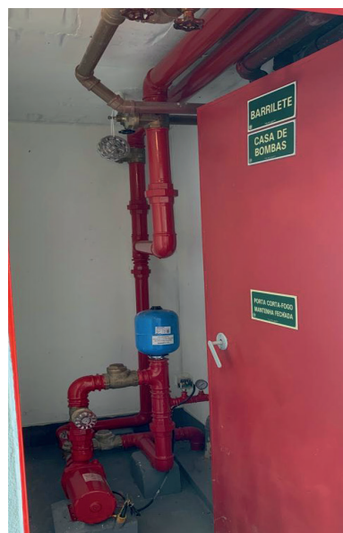
Figura 50 Barrilete, casa de bombas no
