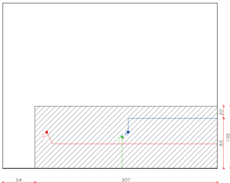
VISTA O1 - VARANDA ESC.: 1/25
