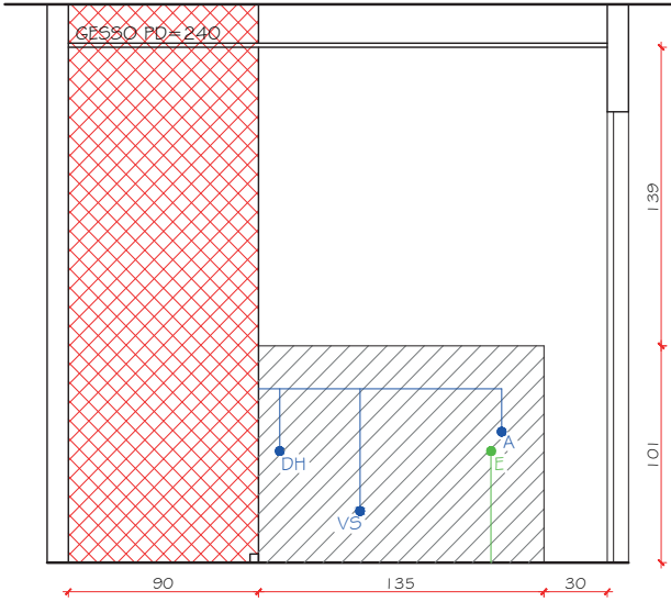
VISTA 01 - BANH SUITE ESC.: 1/25
