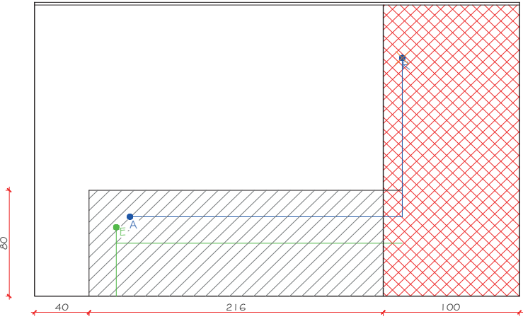
VISTA O I - VARANDA ESC.: 1/25
