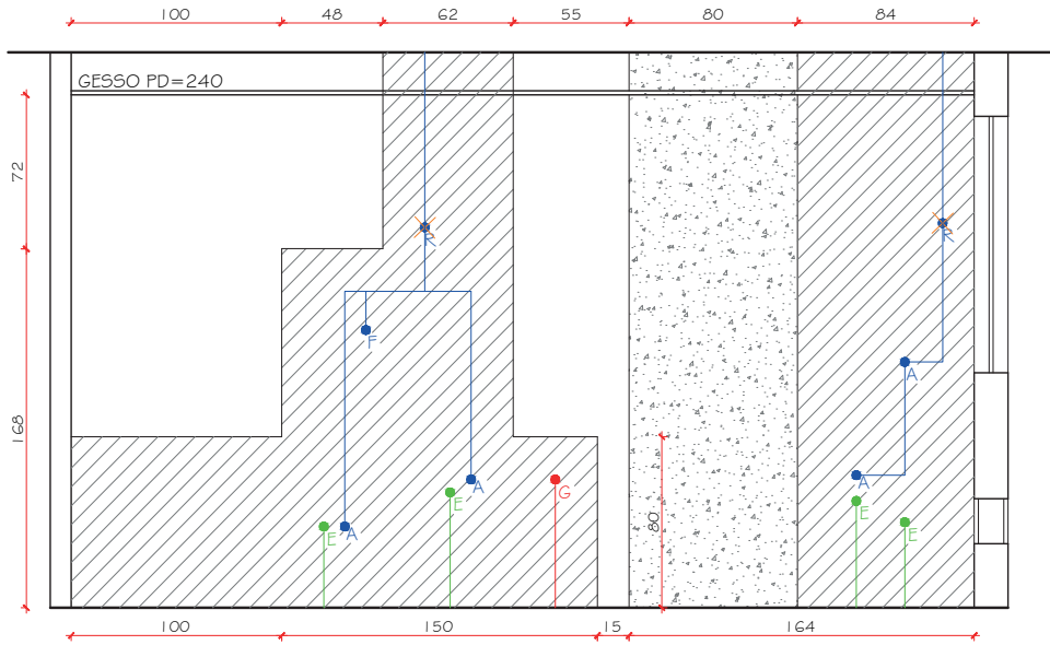
VISTA O1 - COZINHA ESC.: 1/25
