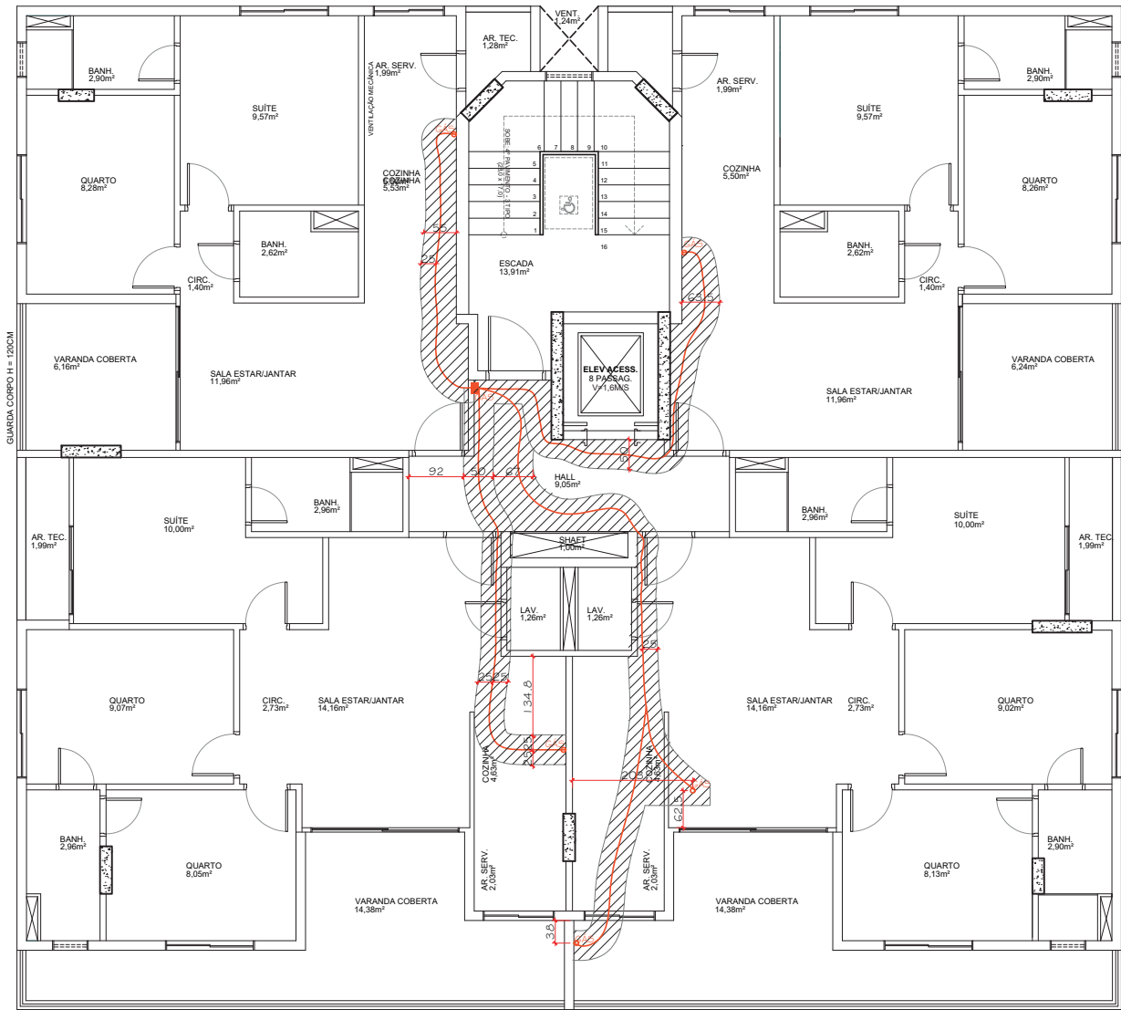
PLANTA BAIXA - TUBULAÇÃO DE GÁS - 5º PAVIMENTO ESC.: 1/50
