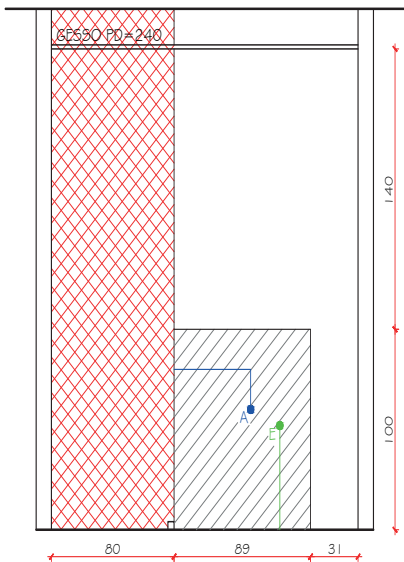
VISTA 01 - BANH SOCIAL ESC.: 1/25
