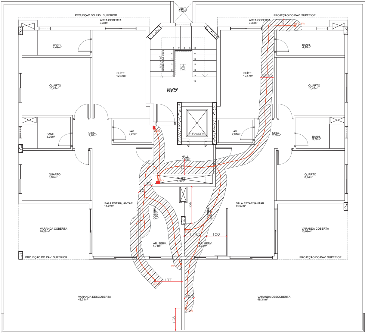
PLANTA BAIXA - TUBULAÇÃO DE GÁS - 6º PAVIMENTO ESC.: 1/50
