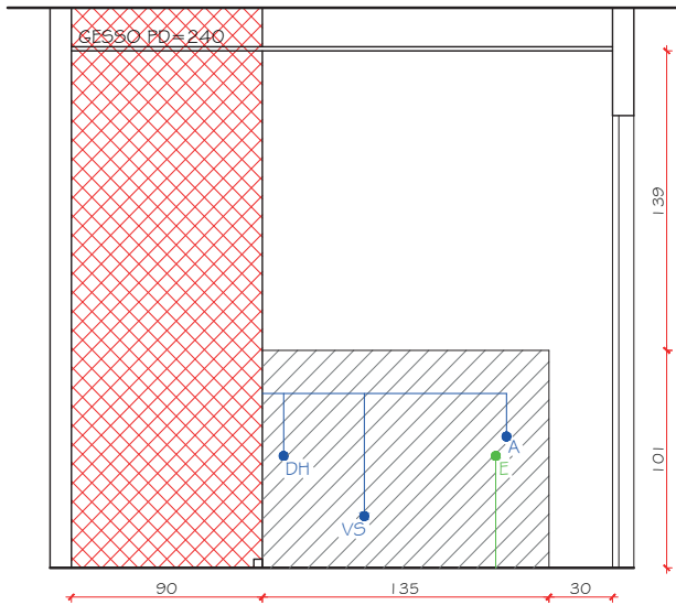
VISTA O1 - BANH SUITE ESC.: 1/25
