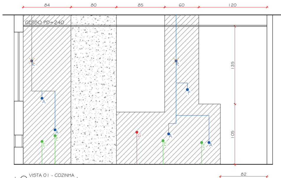
VISTA 01 - COZINHA ESC.: 1/25
