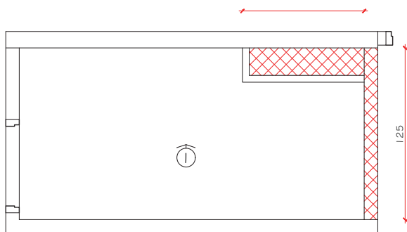
PLANTA BAIXA - BANH SUITE ESC.: 1/25
