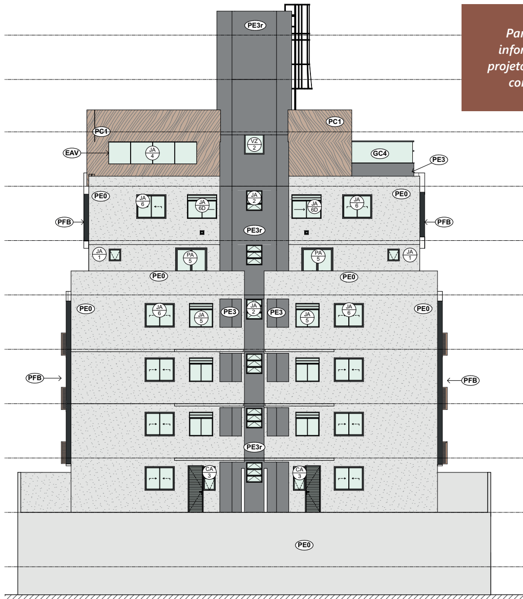
Figura 22 Fachada do Edifício Roof Top com aplicação de Textura e Revestimentos
