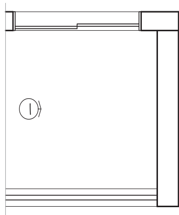
PLANTA BAIXA - VARANDA ESC.: 1/25
