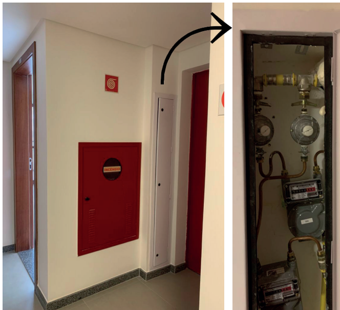
Figura 86 Shaft de gás no hall do pavimento tipo
