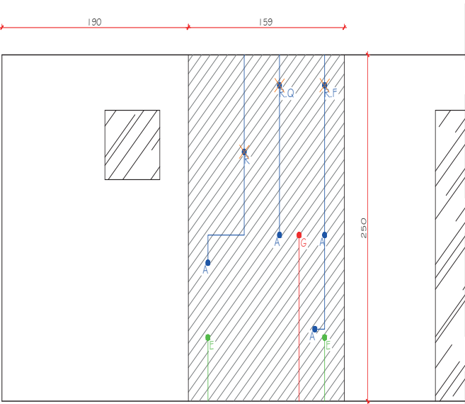
VISTA O.I. - VARANDA FUNDOS ESC.: 1/25
