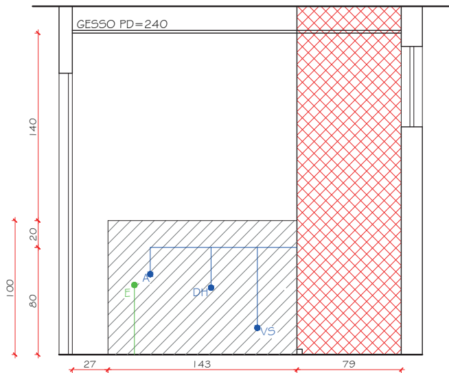
VISTA 01 - BANH SUITE ESC.: 1/25
