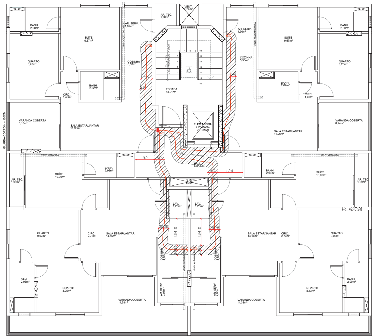
PLANTA BAIXA - TUBULAÇÃO DE GÁS - 3º PAVIMENTO ESC.: 1/50
