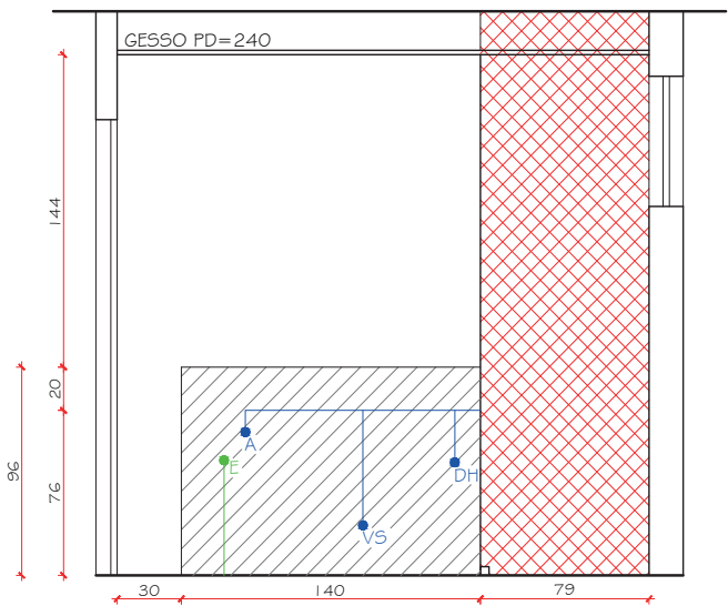
VISTA O.I. - BANH SOCIAL ESC.: 1/25
