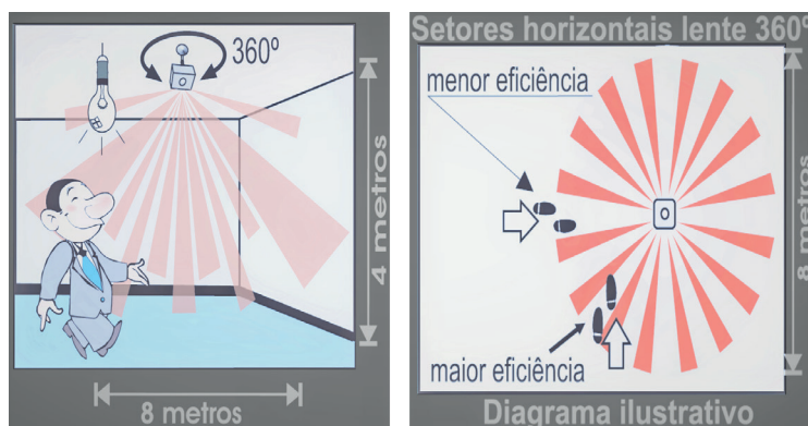
Figura 79 área de abrangência de Sensor de presença do modelo Qa19 Bivolt
