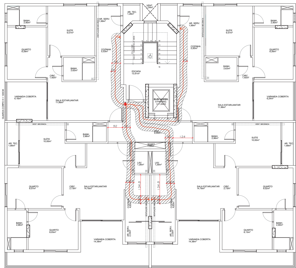
PLANTA BAIXA - TUBULAÇÃO DE GÁS - 4º PAVIMENTO ESC.: 1/50
