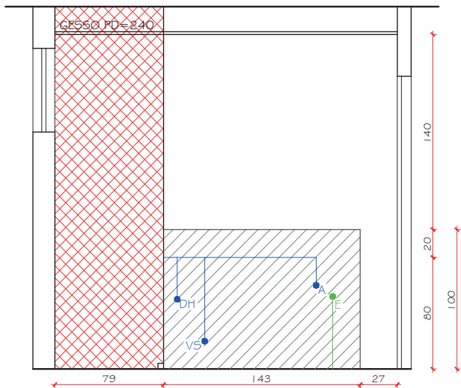
VISTA O.I - BANH SUITE Esc.: 1/25
