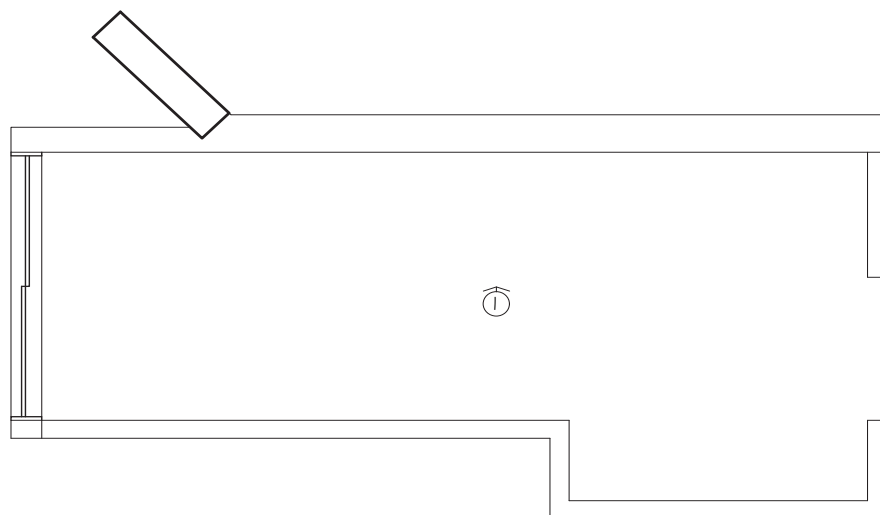
PLANTA BAIXA - COZINHA ESC.: 1/25
