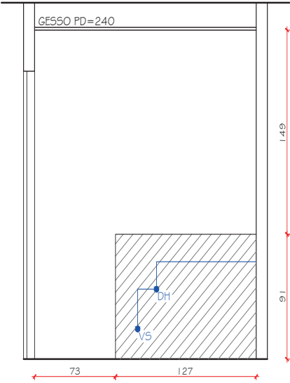
VISTA 02 - BANH SOCIAL ESC.: 1/25
