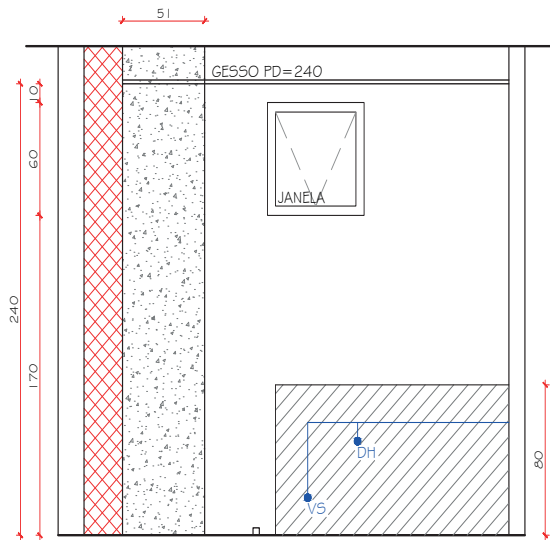
VISTA 02 - BANH SUÍTE ESC.: 1/25
