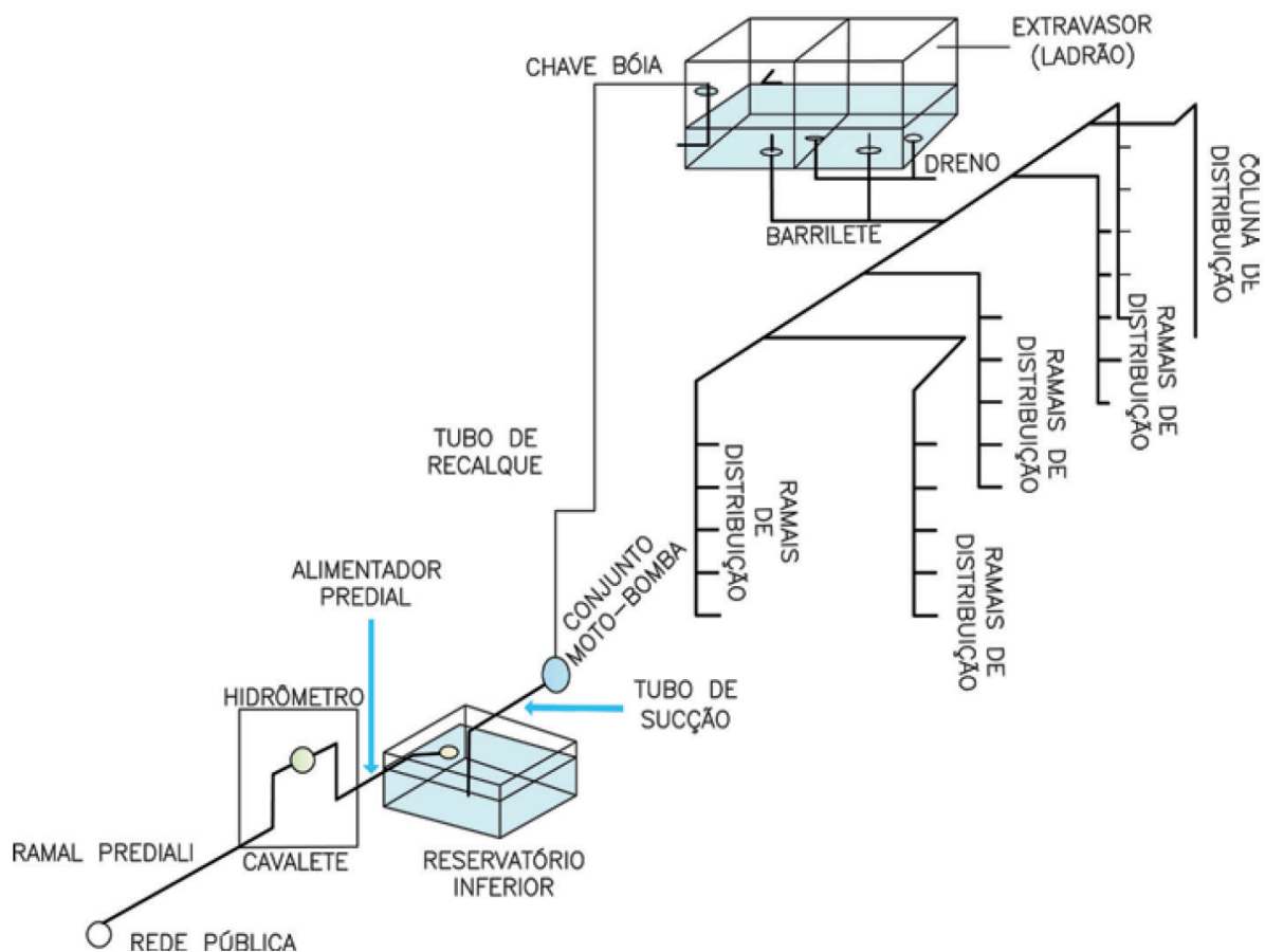
Figura 47 Representação esquemática do sistema de distribuição de água potável do edifício
