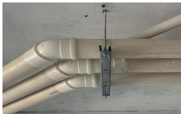
Figura 56 Suportes da tubulação presa ao teto
