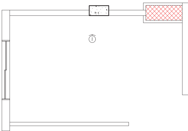
PLANTA BAIXA - COZINHA ESC.: 1/25
