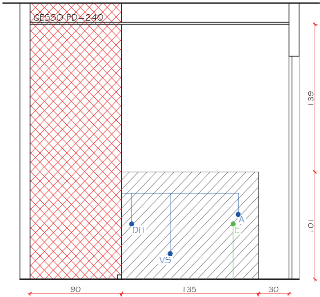
VISTA O1 - BANH SUITE ESC.: 1/25
