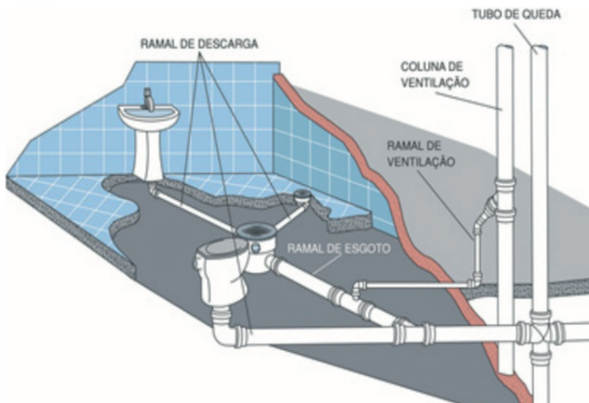
Figura 53 Representação do sistema de água não potável de um banheiro
