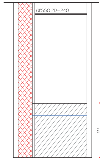
VISTA 03 - BANH SOCIAL ESC.: 1/25
