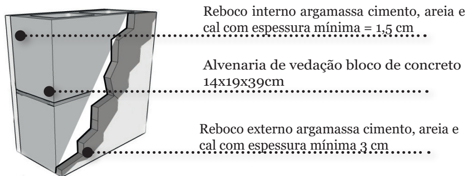
Quadro 2 Camadas que compõe o sistema de vedação
