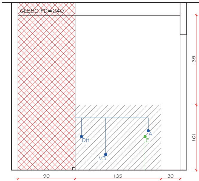
VISTA 01 - BANH SUITE ESC.: 1/25
