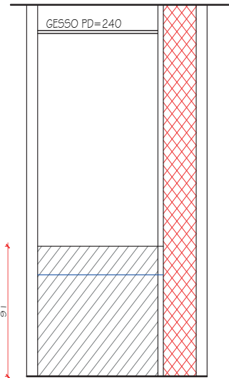
VISTA 03 - BANH SOCIAL ESC.: 1/25
