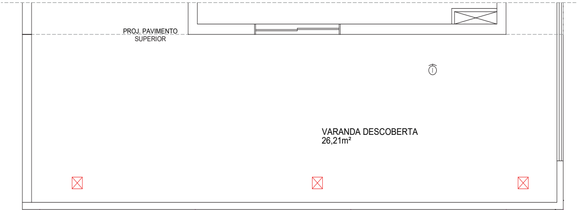
PLANTA BAIXA - VARANDA DESCOBERTA 202 ESC.: 1/25
