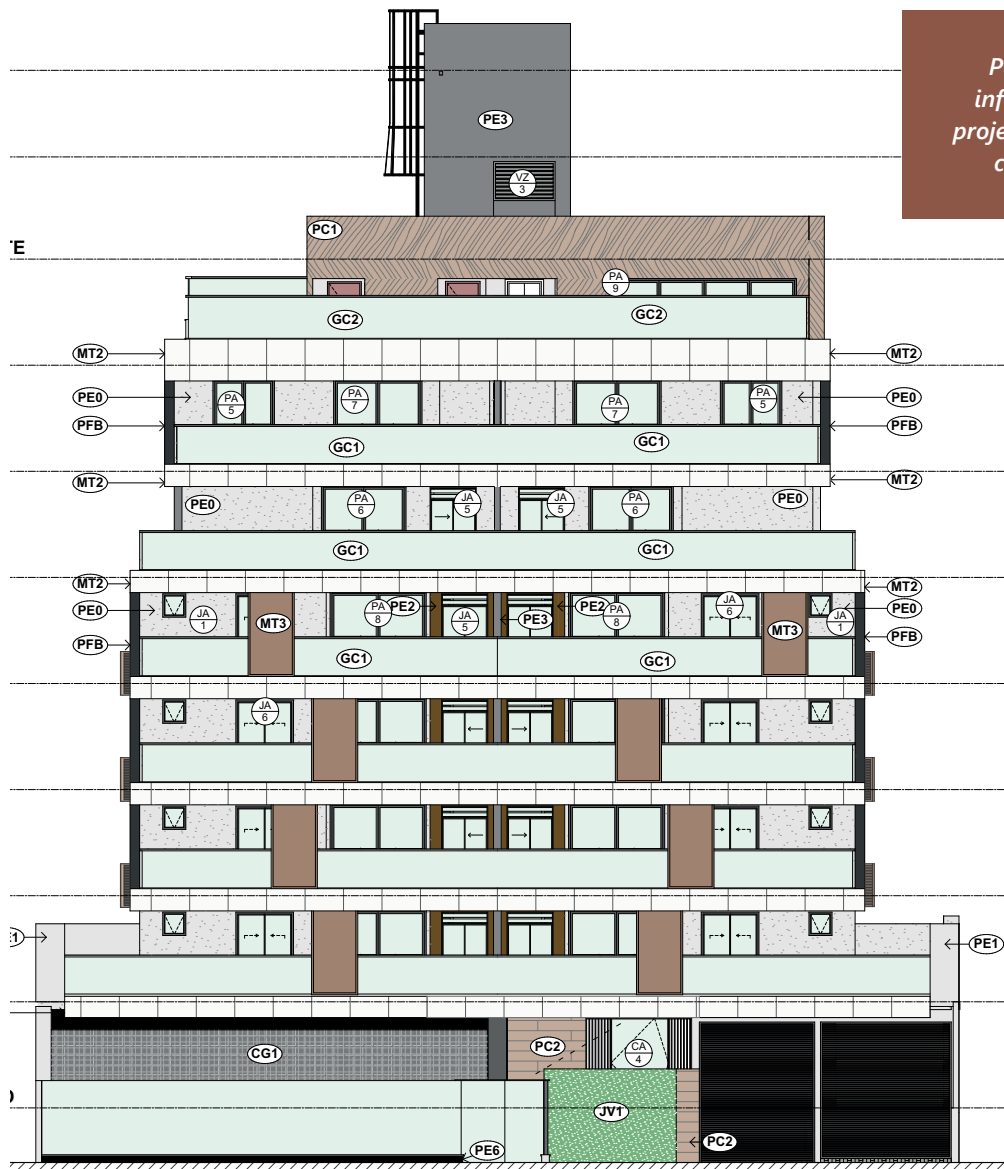
Figura 20 Fachada Principal do Edifício Roof Top com aplicação de Textura e Revestimentos
